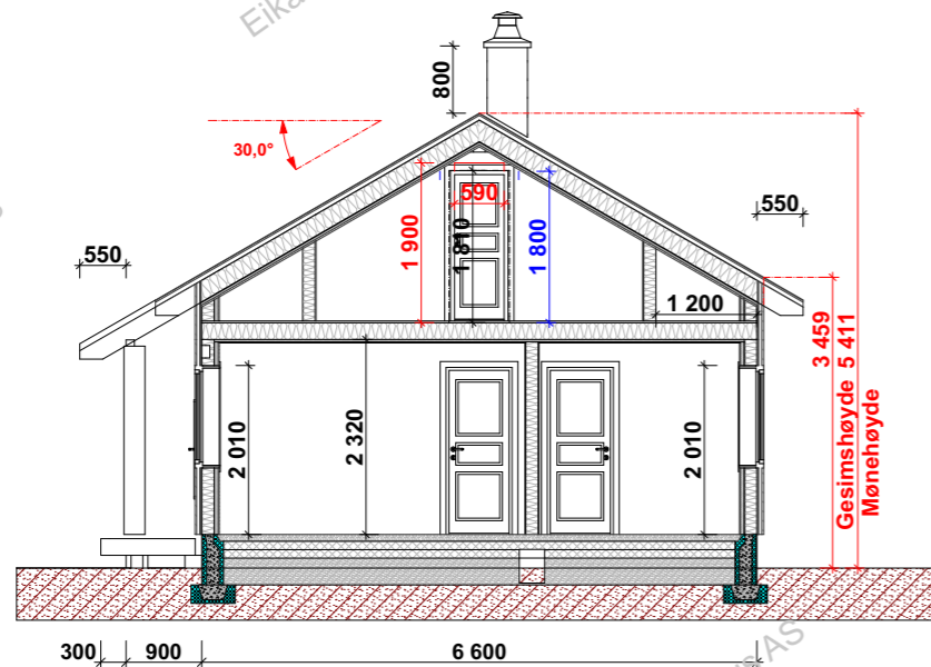
Snitt A-A
