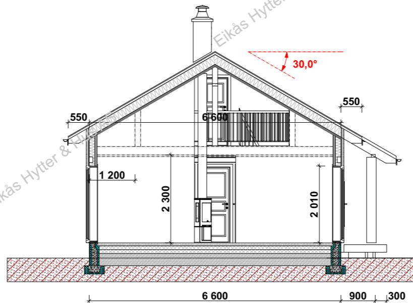
Snitt B-B
