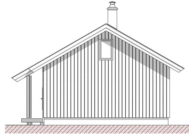
Fasade mot
