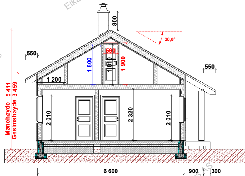
Snitt A-A
