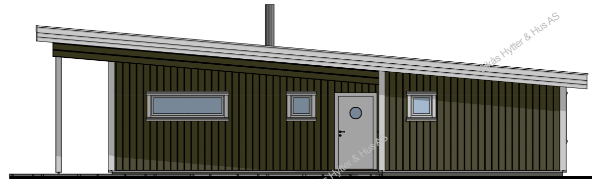
Fasade mot
