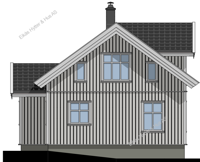
Fasade mot
