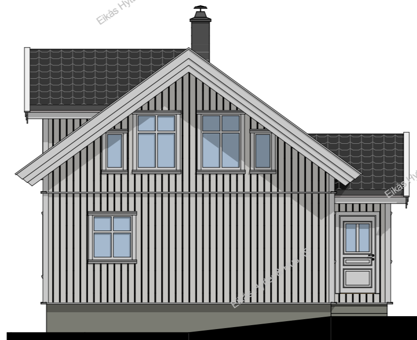
Fasade mot
