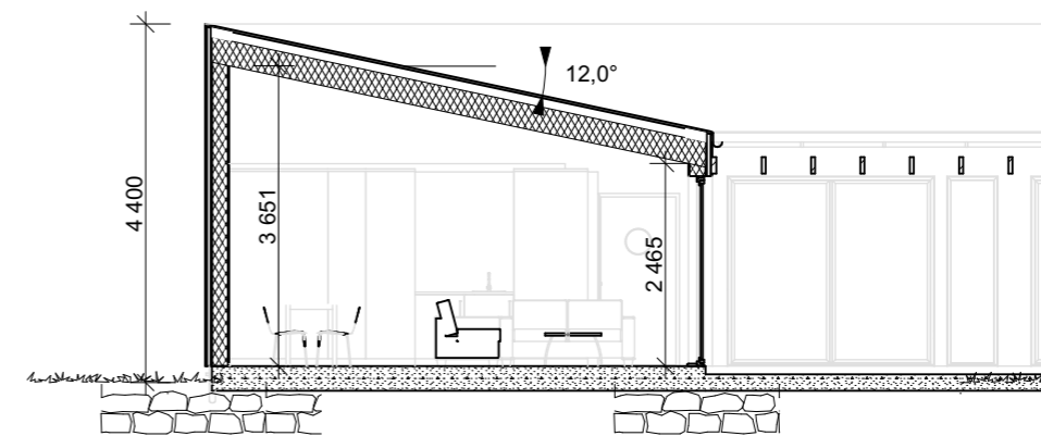
Snitt A-A
