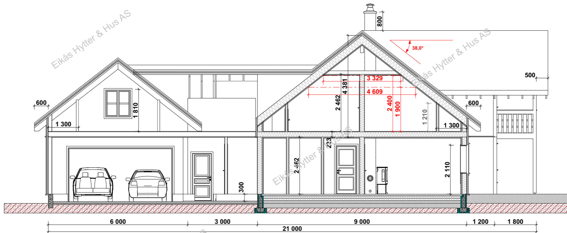
Snitt A-A
