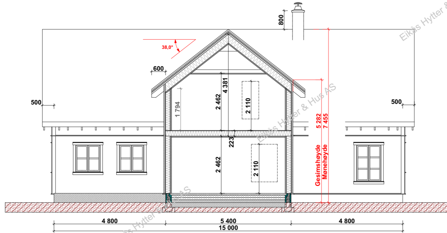
Snitt B-B
