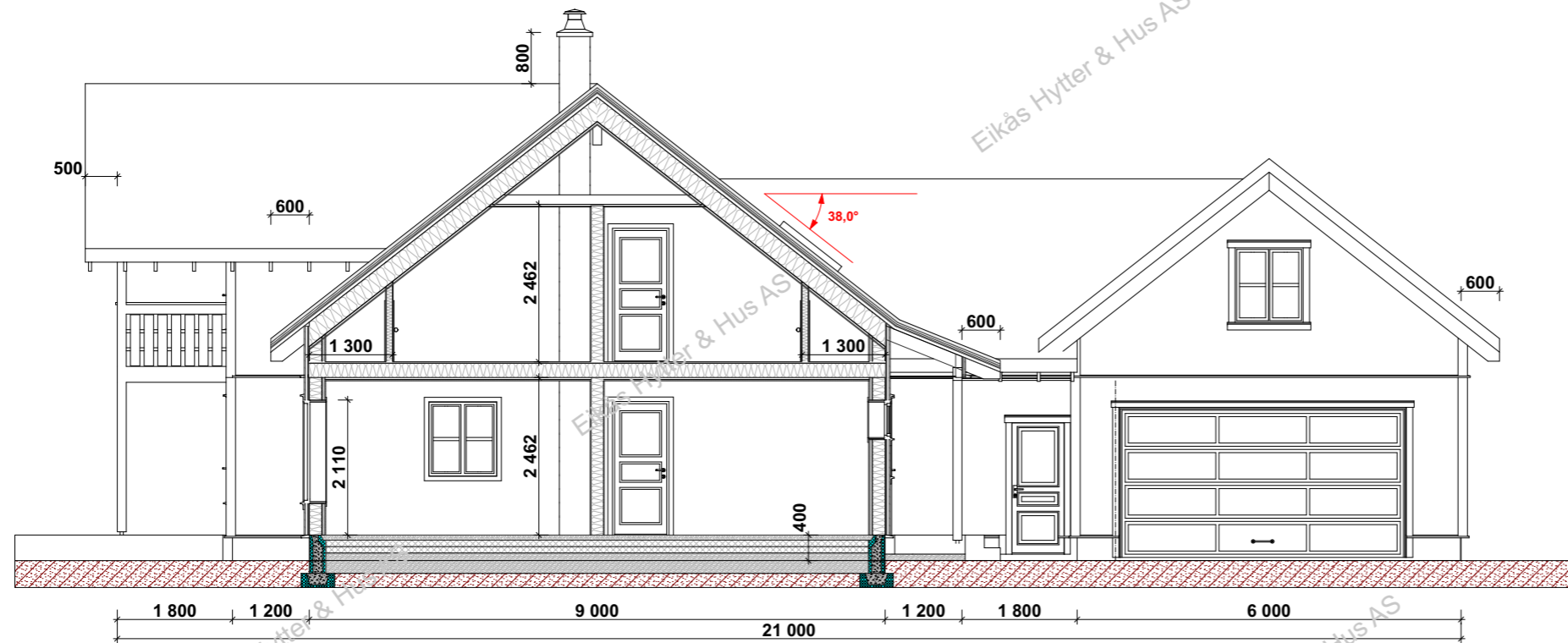
Snitt C-C
