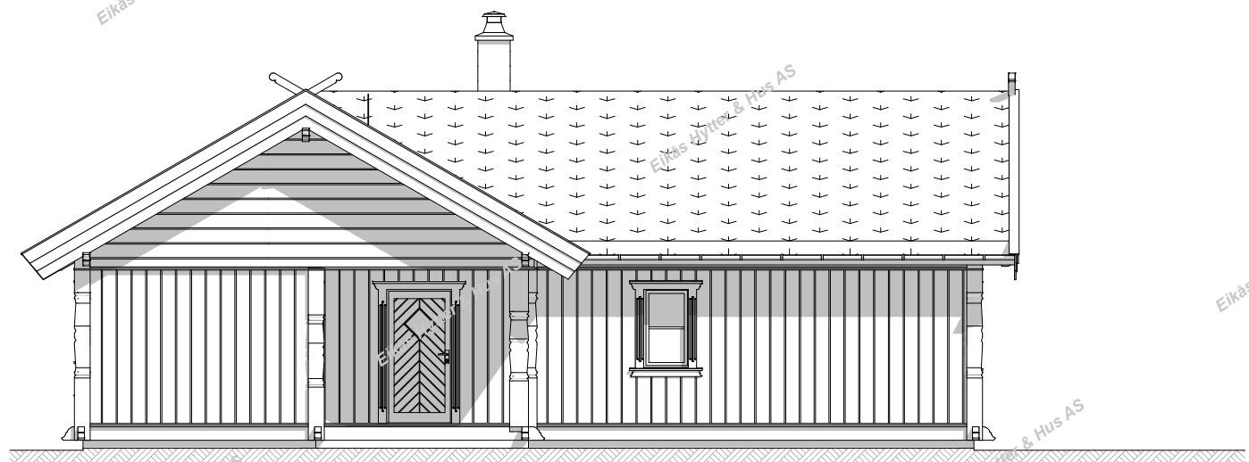
Fasade 3
