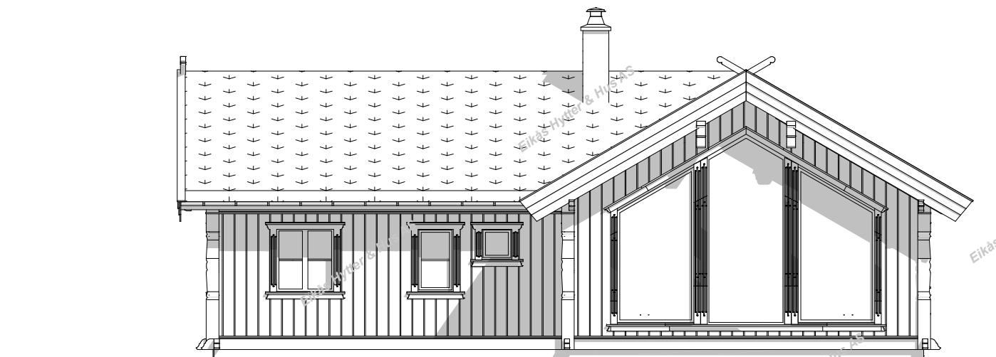
Fasade 1
