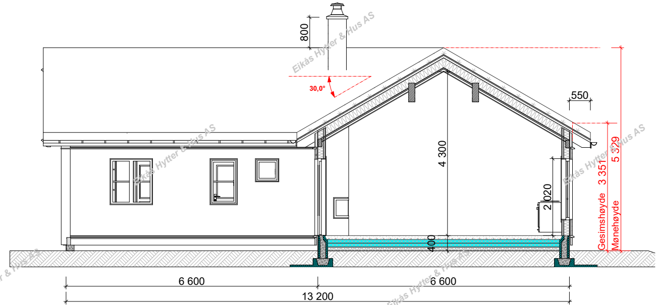
Snitt B-B
