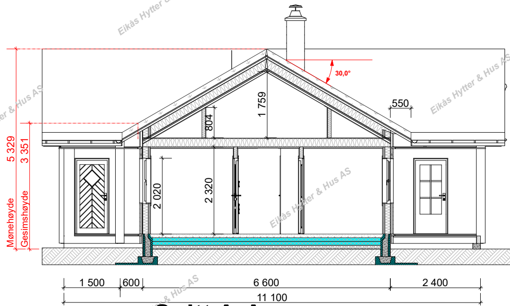
Snitt A-A
