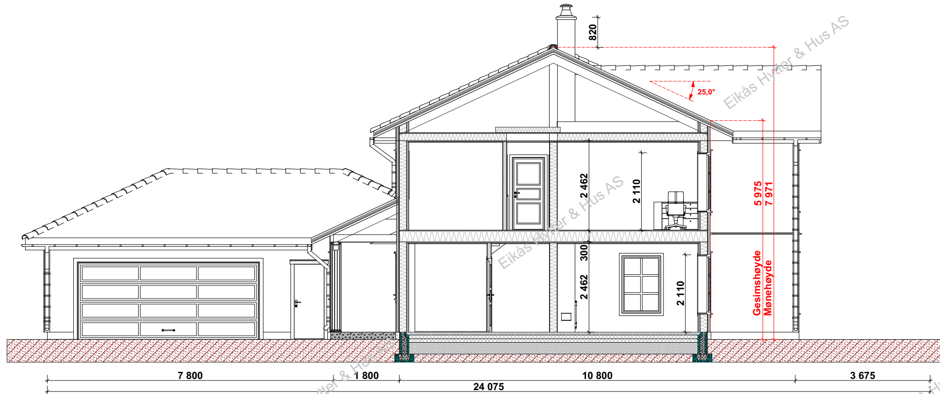
Snitt A-A
