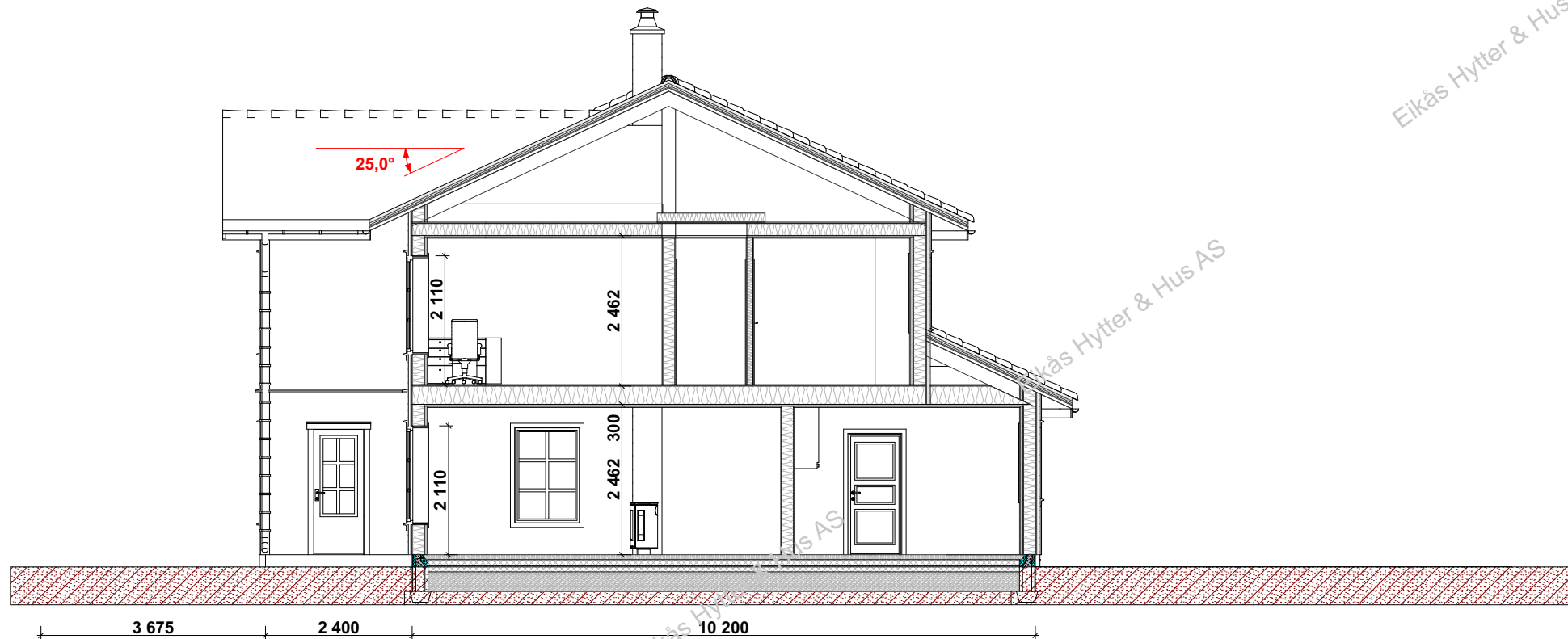
Snitt C-C
