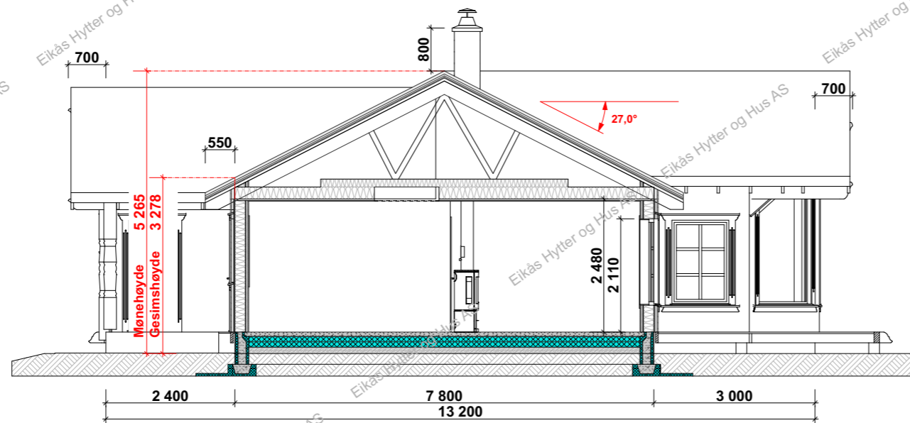
Snitt A:A
