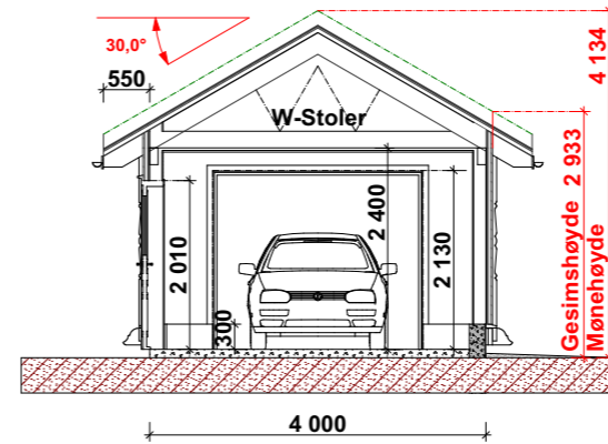
Snitt A-A
