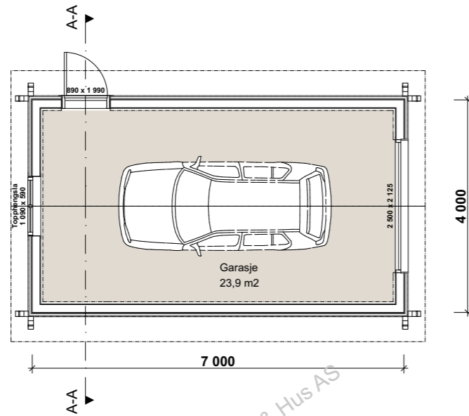
Hovedplan
